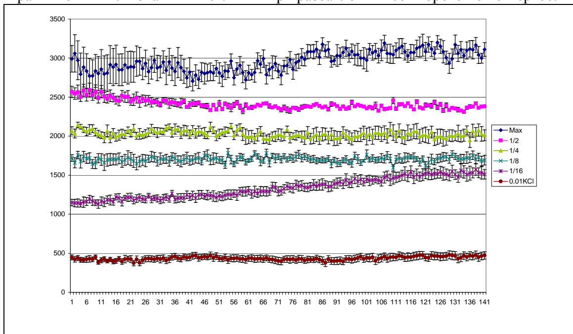
Рис.1. Временная зависимость площади засветки от концентраций раствора полиокса.
